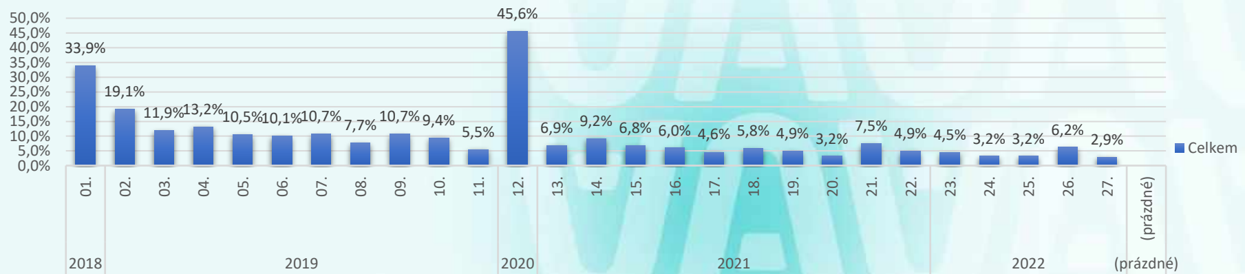
Phishingové kampaně 2018 - 2022
